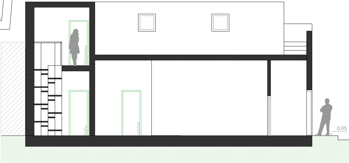
SECCION 1-1
